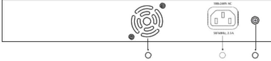
Şekil 1-2 BDCOM S2210PB anahtarının arka şablonu
